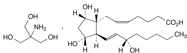
Figure B-3-8. – Dinoprost trometamol (1312)
